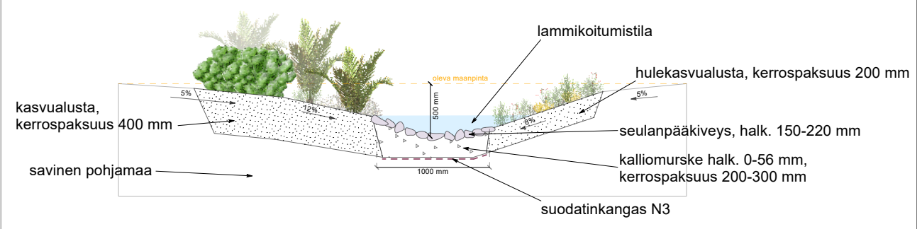
det2. Kosteikkoistutus, periaatepoikkileikkaus 1:50
