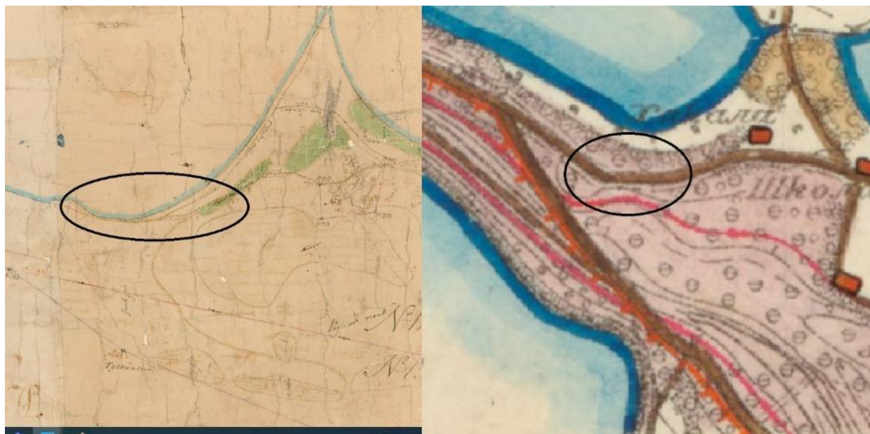
Kuva 35. Kylien välinen tielinjaus Heponiemen 1700-luvun isojakokartalla (vas.) ja 1800-luvun senaatinkartalla.
