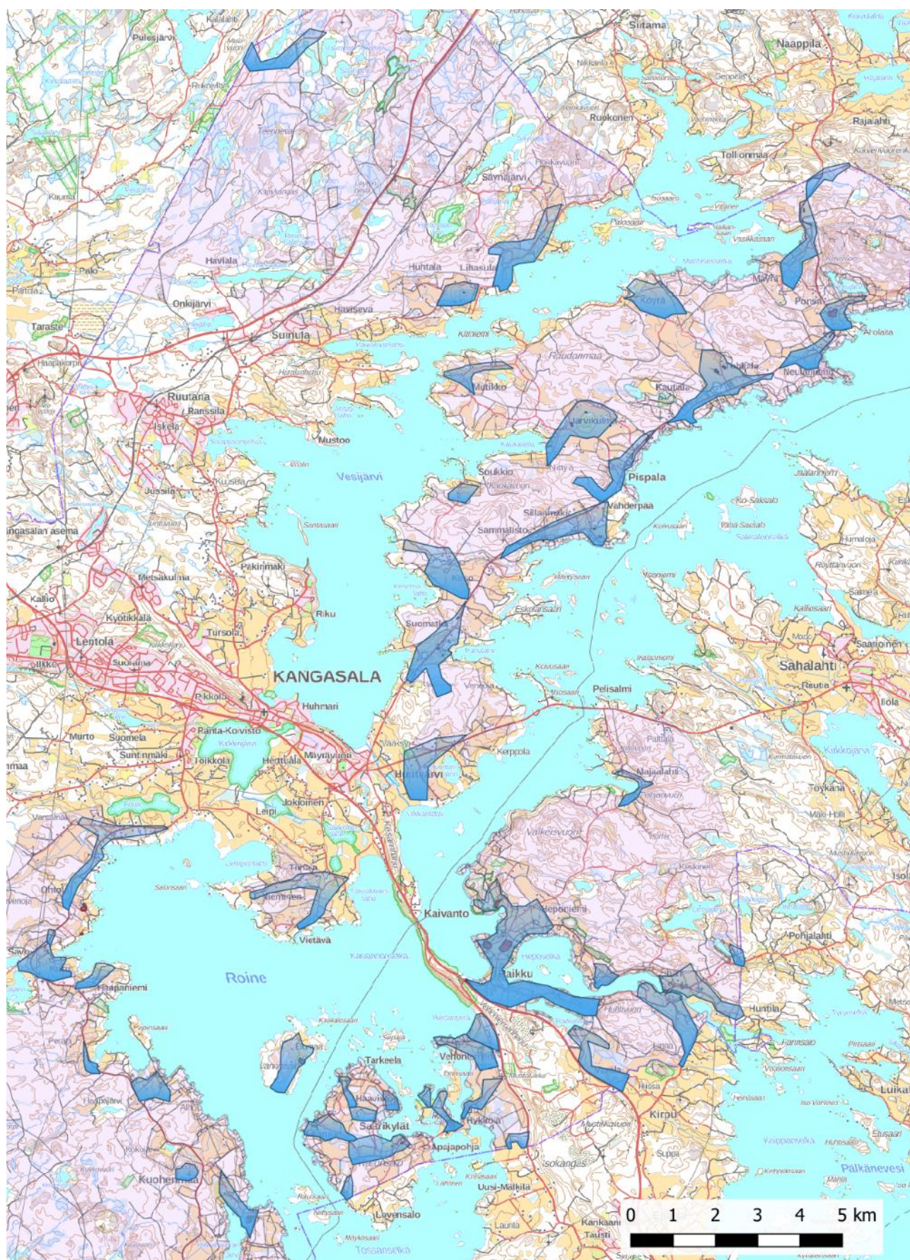
Kartta 3. Maastossa tarkastetut alueet merkitty karttaan sinisellä. MK 1:100 000.
