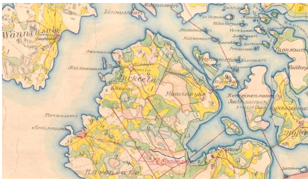
Kuva 87. Pitäjänkartta Saarikylästä ja Vänninsalosta.
