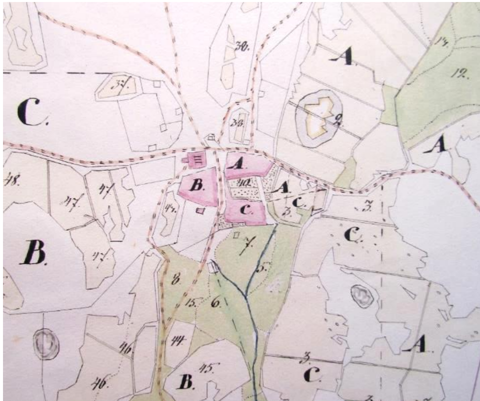
Kuva 70. Kautialan kylä Pispalan isojakokartalla.
