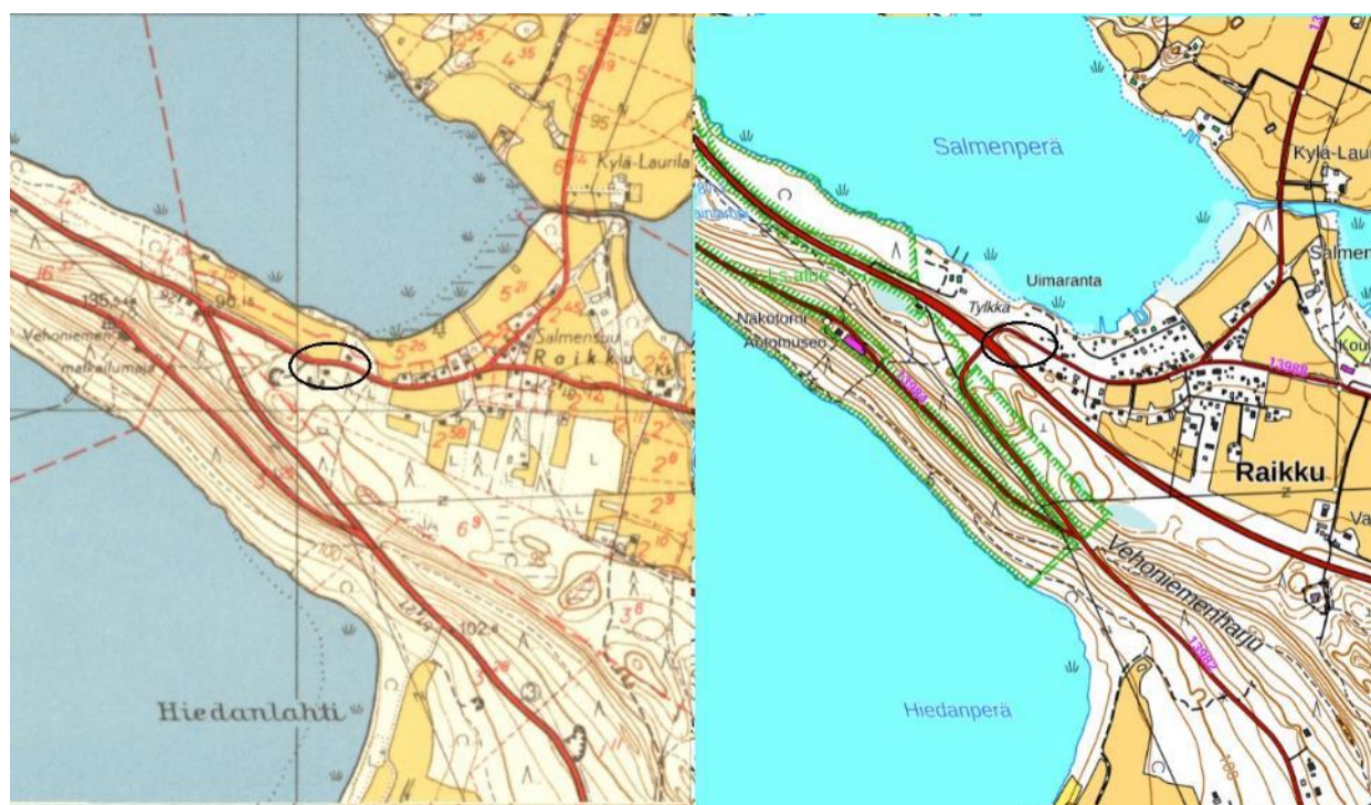
Kuva 36. Muuttunut tielinjaus 1953 peruskartalla (vas.) ja nykykartalla.
