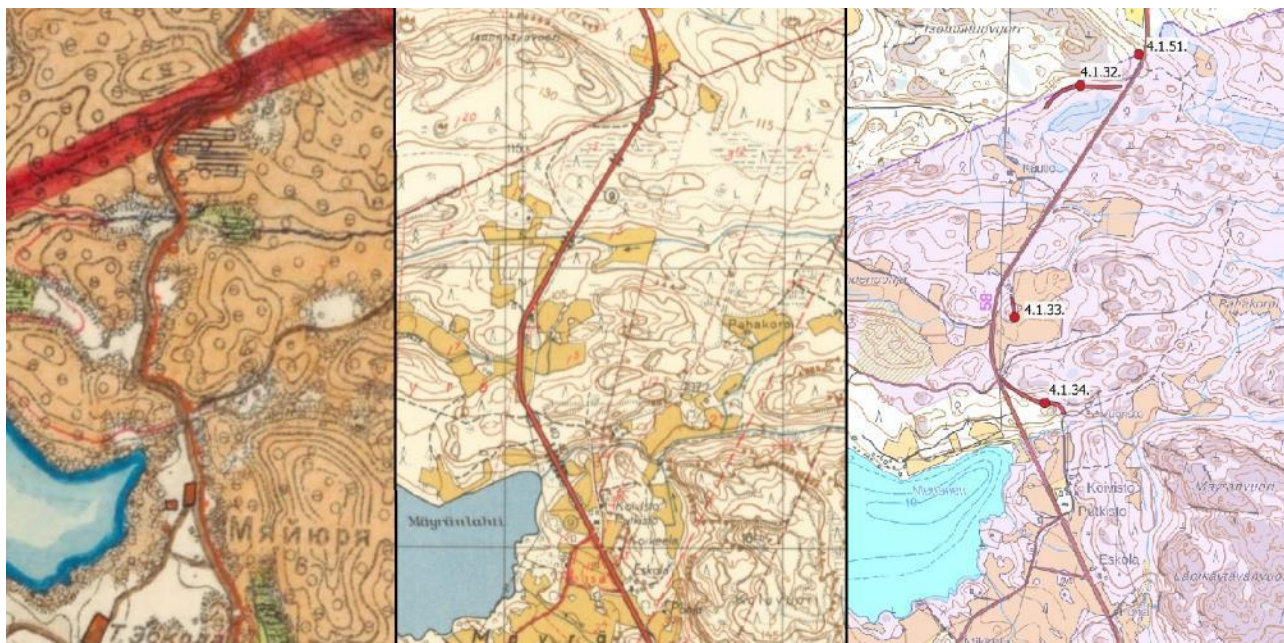
Kuva 23. Vanha tielinja näkyy vielä senaatinkartalla (vas.). Vuoden 1954 painetulla kartalla näkyy jo uusi tielinja. Oikealla uusi maastokartta ja pois käytöstä jääneet tielinjaukset.
