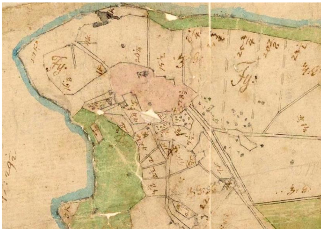
Kuva 76. Keljon kylätontti punaisella Heponiemen isojakokartassa vuodelta 1774.
