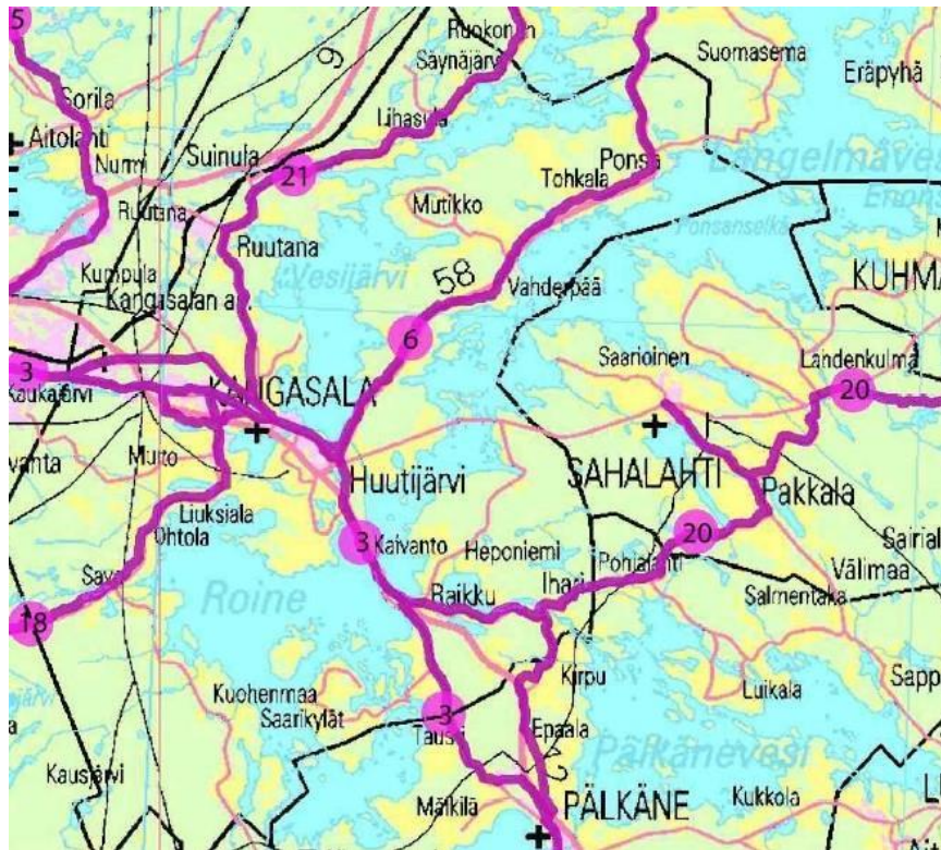
Kuva 1. Ote Kalle Luodon laatimasta Pirkanmaan historiallisesti merkittävät tielinjaukset- raportista (2011). Inventoinnissa kiinnitettiin huomiota etenkin teihin nro 6 (Kangasala-Orivesi), 3 (Tampere-Pälkäne-Hämeenlinna) ja 20 (Pälkäne-Sahalahti-Kuhmalampi).
