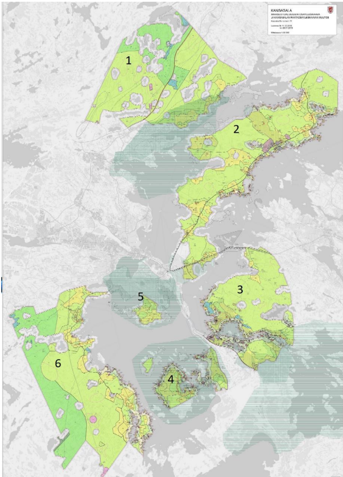
Kartta 1. Lähestymiskartta. Kangasalan kunnan laatima kartta osayleiskaavainvoinnin alueista. Alueiden numerointi on tehty inventoinnin kenttätöitä varten. Ei mittakaavassa.
