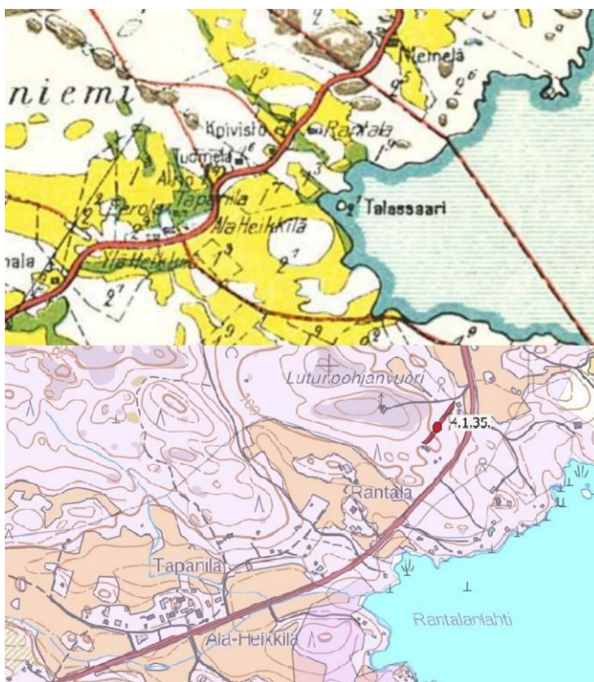
Kuva 31. Yllä Kangasalan kartta 1930-luvulta, jossa näkyy alkuperäinen tielinjaus. Alla nykykartta ja Rantalan kohdalla pois käytöstä jäänyt tielinjaus.
