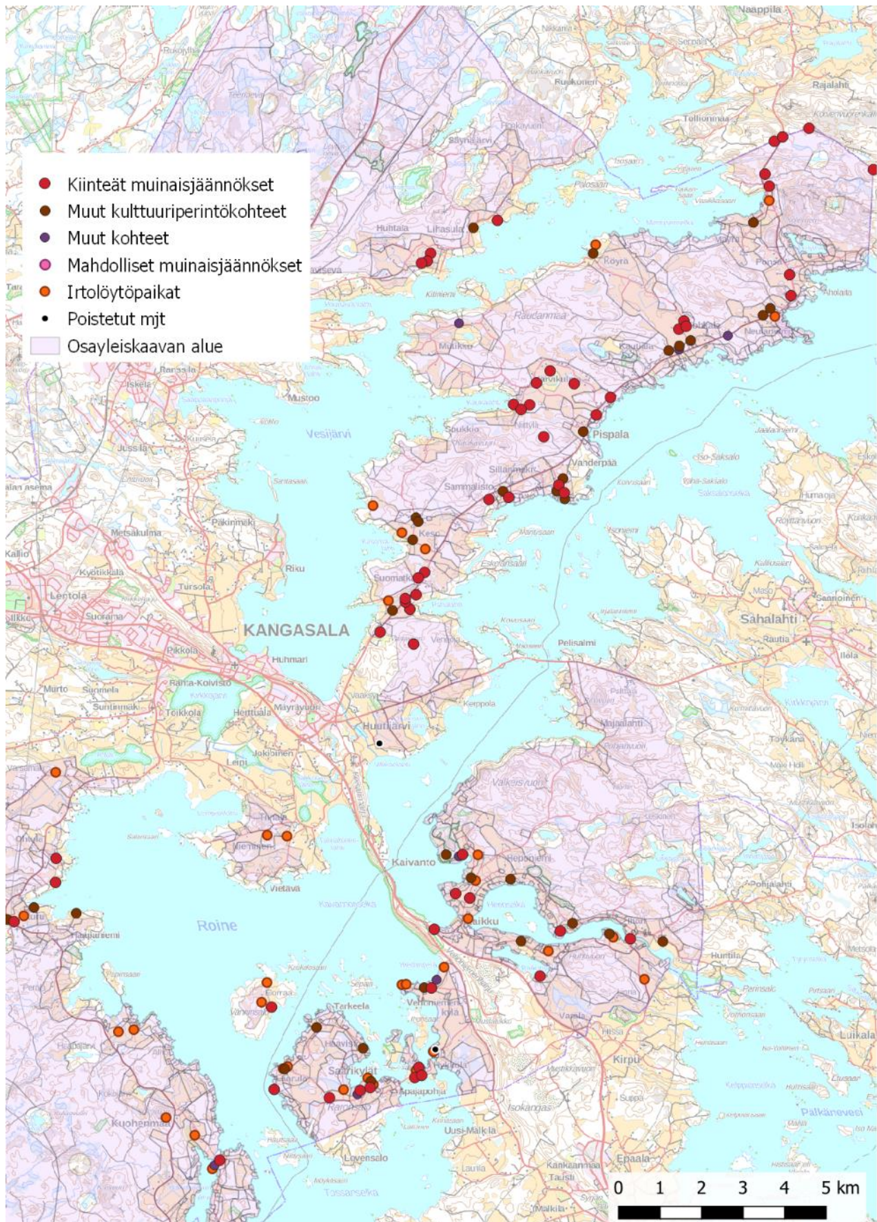
Kartta 2. Inventointialue ja muinaisjäännöskohteiden sijoittuminen kaavoitettavalle alueelle. MK1:100 000.
