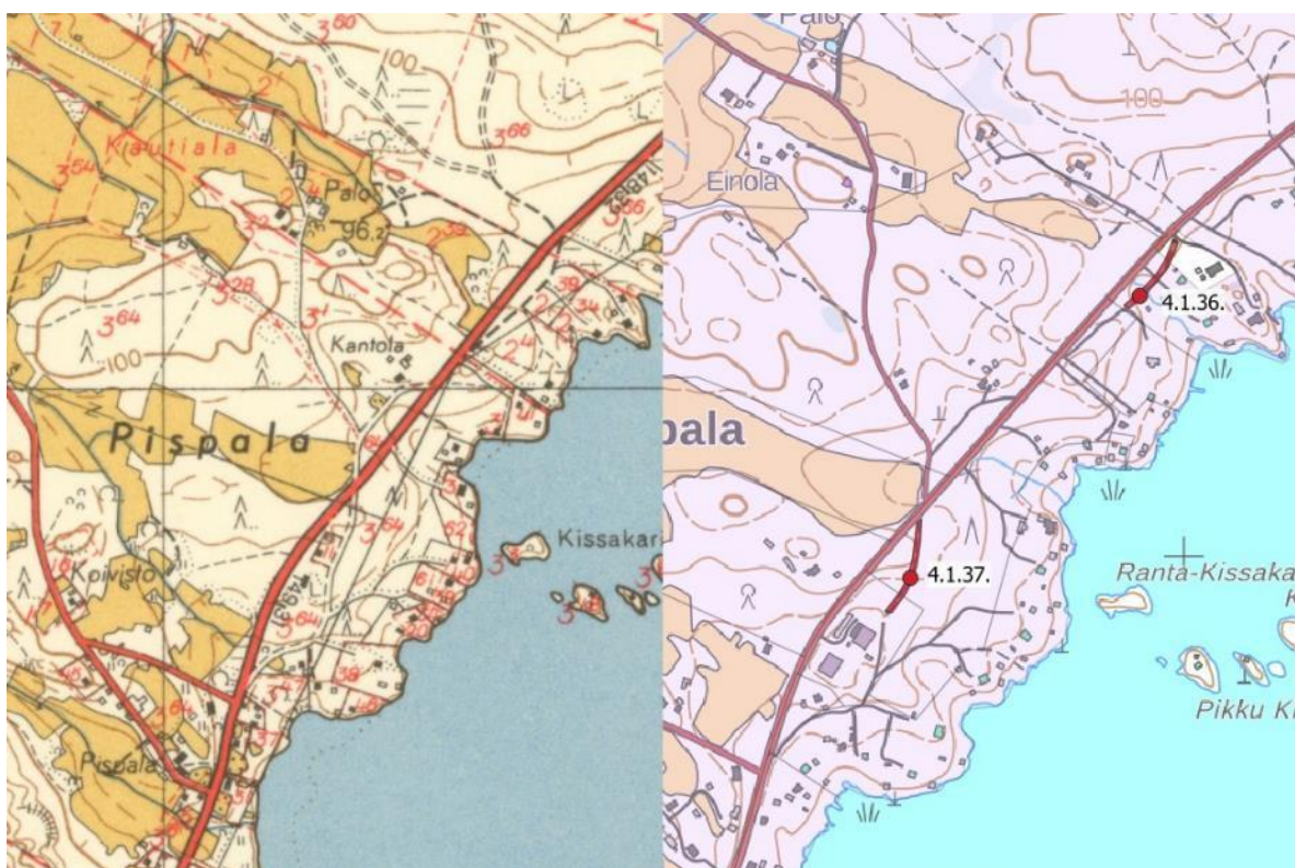
Kuva 33. Vasemmalla vuoden 1954 painettu kartta, jossa vanha tielinjaus on jäänyt pihatieksi ja metsäpoluksi. Oikealla pois käytöstä jääneet tielinjaukset nykykartalla.
