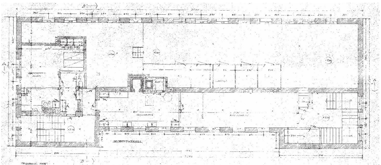
Ullakkokerroksen pohjapiirustus vuodelta 1952. Ullakko on pääosin varastotilaa, minkä lisäksi siellä on keittiö, ruokailuhuone sekä vahtimestarin asunto.
