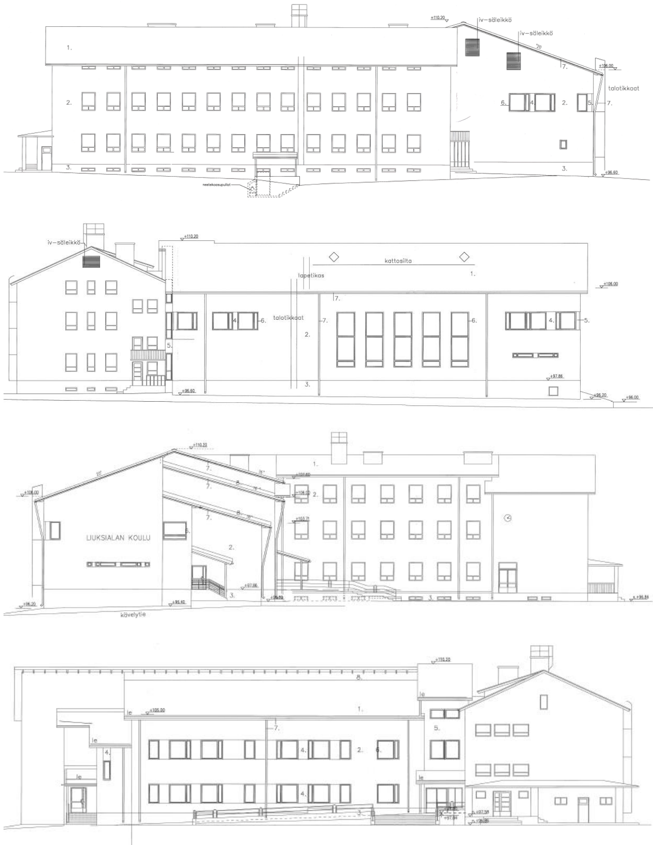
Liuksialan koulurakennuksen laajennusosan julkisivupiirustukset itään, pohjoiseen, länteen ja etelään (ylhäältä alas) vuodelta 2005.
