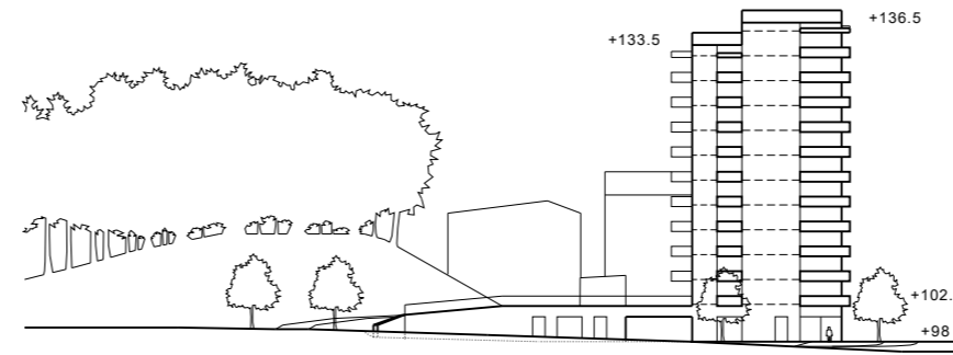
Katujulkisivu Kunnantielle
