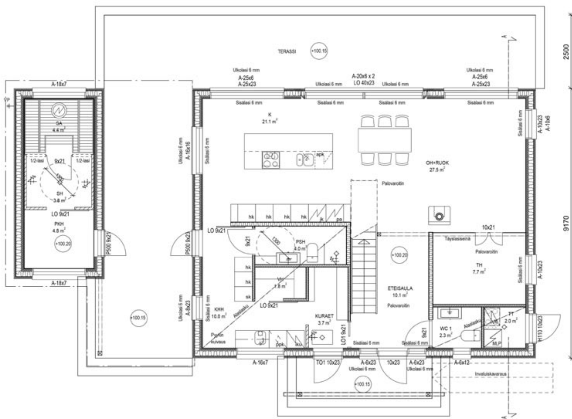
Pohjapiirros 1. krs.
